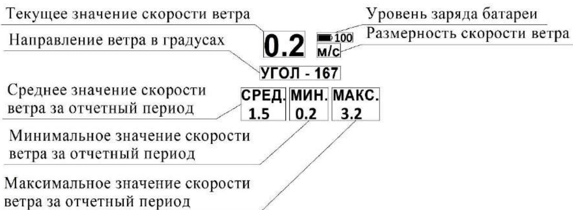
Рисунок 1 Внешний вид и габаритные размеры изделия
